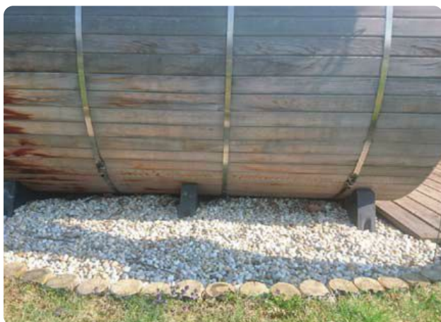
Štrkové lôžko s betónovými podperami
